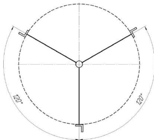
Рисунок 1 – Схема размещения растяжек в плане
